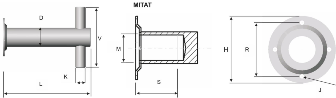
TALUKKO 2. Valuankkureiden mitat [mm].
